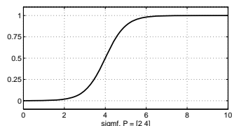
sigmf
