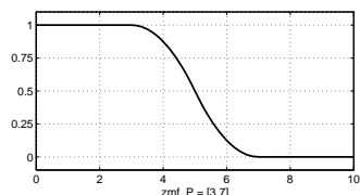
zmf
